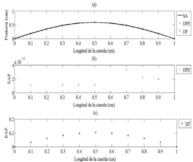
FIGURA 3. (a) Movimiento de una cuerda de un 1 cm de longitud para t=0.3 seg, \Delta x = 0.1 cm y \sigma = 3/4 . (b) Error absoluto porcentual de la solución del esquema de diferencias finitas exactas. (c) Error absoluto porcentual de la solución del esquema de diferencias finitas.
